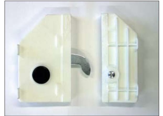
1070380 + 107F380. Gancio maschio e femmina non universali / Not universal male and female fastener
