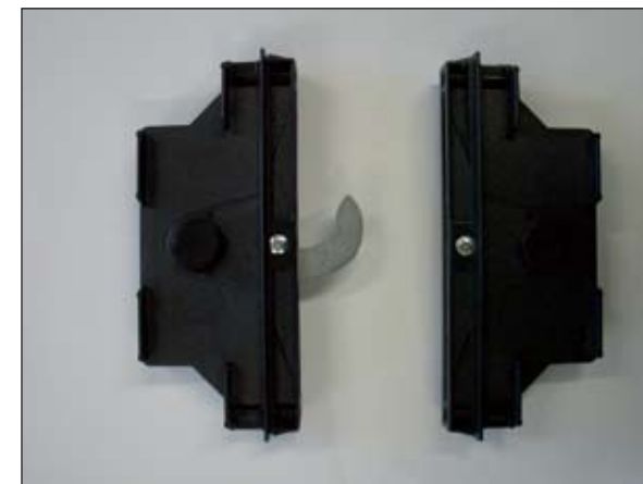
1070078. Gancio maschio universale / Male universal fastener
