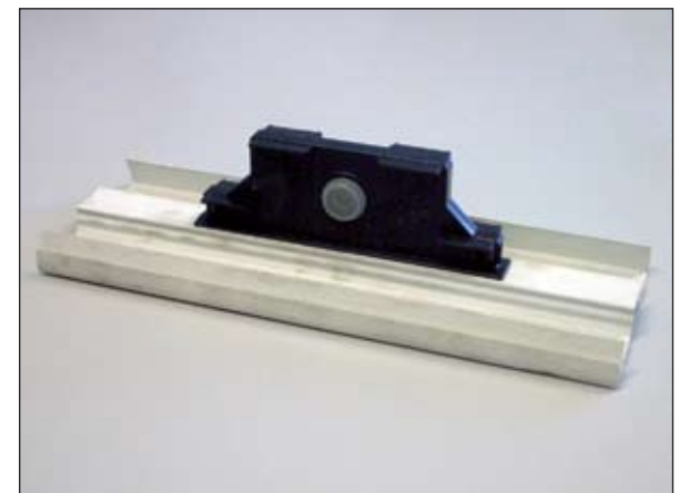
1070078. Gancio maschio universale con battuta per profilo in plastica / Male universal fastener for plastic profile.
